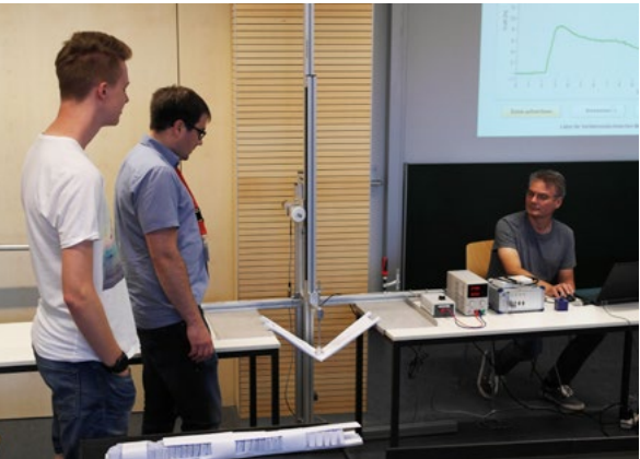
Abb. 81: Belastungstest Papierbrücke
