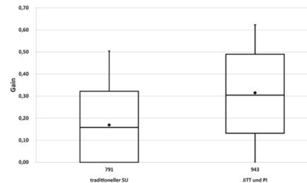
Abb. 63: Boxplot
